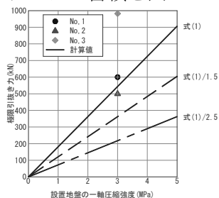
図. 10 試験値と計算値の対比 (P200)
