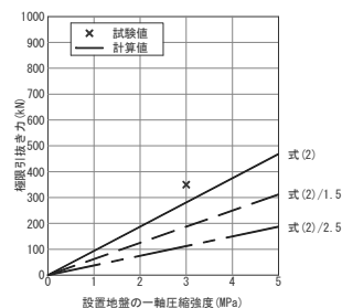
図. 11 試験値と計算値の対比 (P150)
