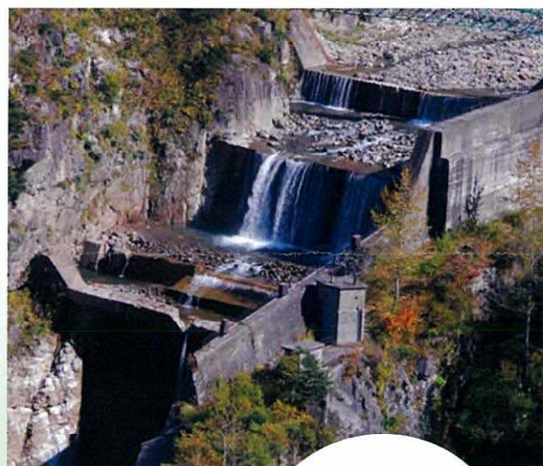
白岩砂防堰堤 (重要文化財)
